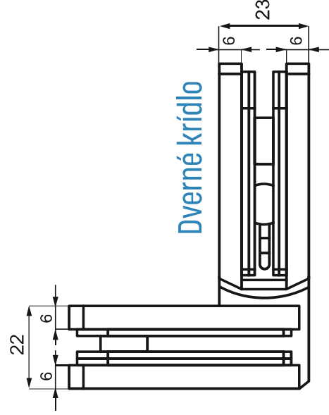
Bočný diel
