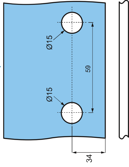
Bočný diel
